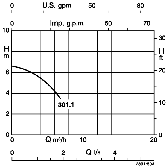
Überflur-Box Normalausführung n = 2800 1/min
