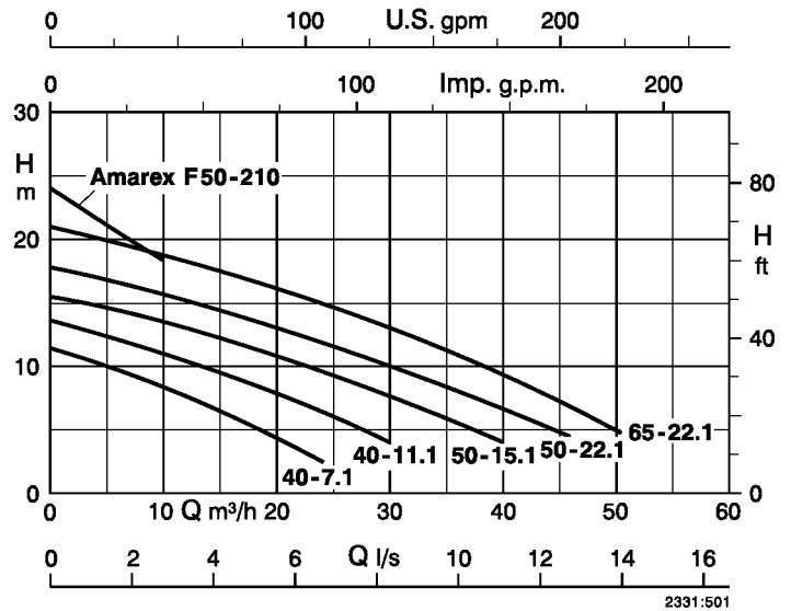
Überflur-Box Ausführung R n = 2800 1/min
